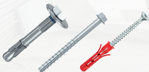
Mechanische ankers
