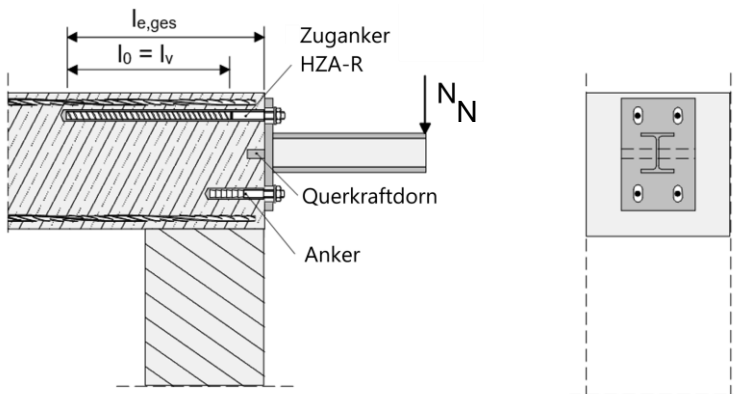
Bild A8: Übergreifungsstoß für die Verankerung von auskragenden Bauteilen
