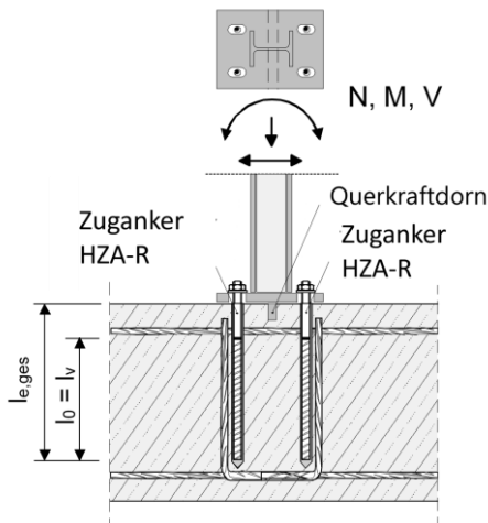
Bild A8: Übergreifungsstoß für die Verankerung von auskragenden Bauteilen
